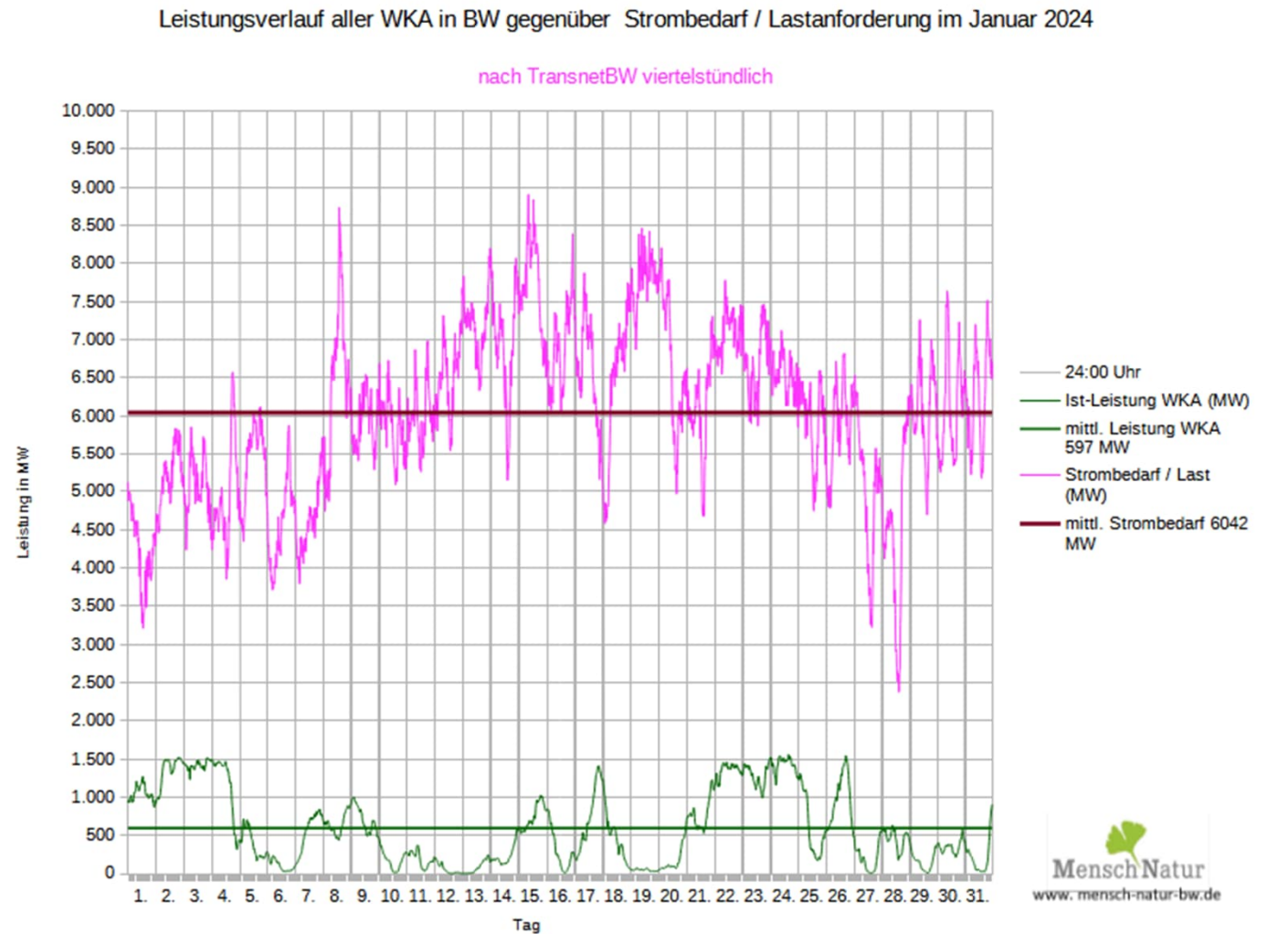
Leistungsverlauf Windleistung gegen Strombedarf (Last) TransnetBW
